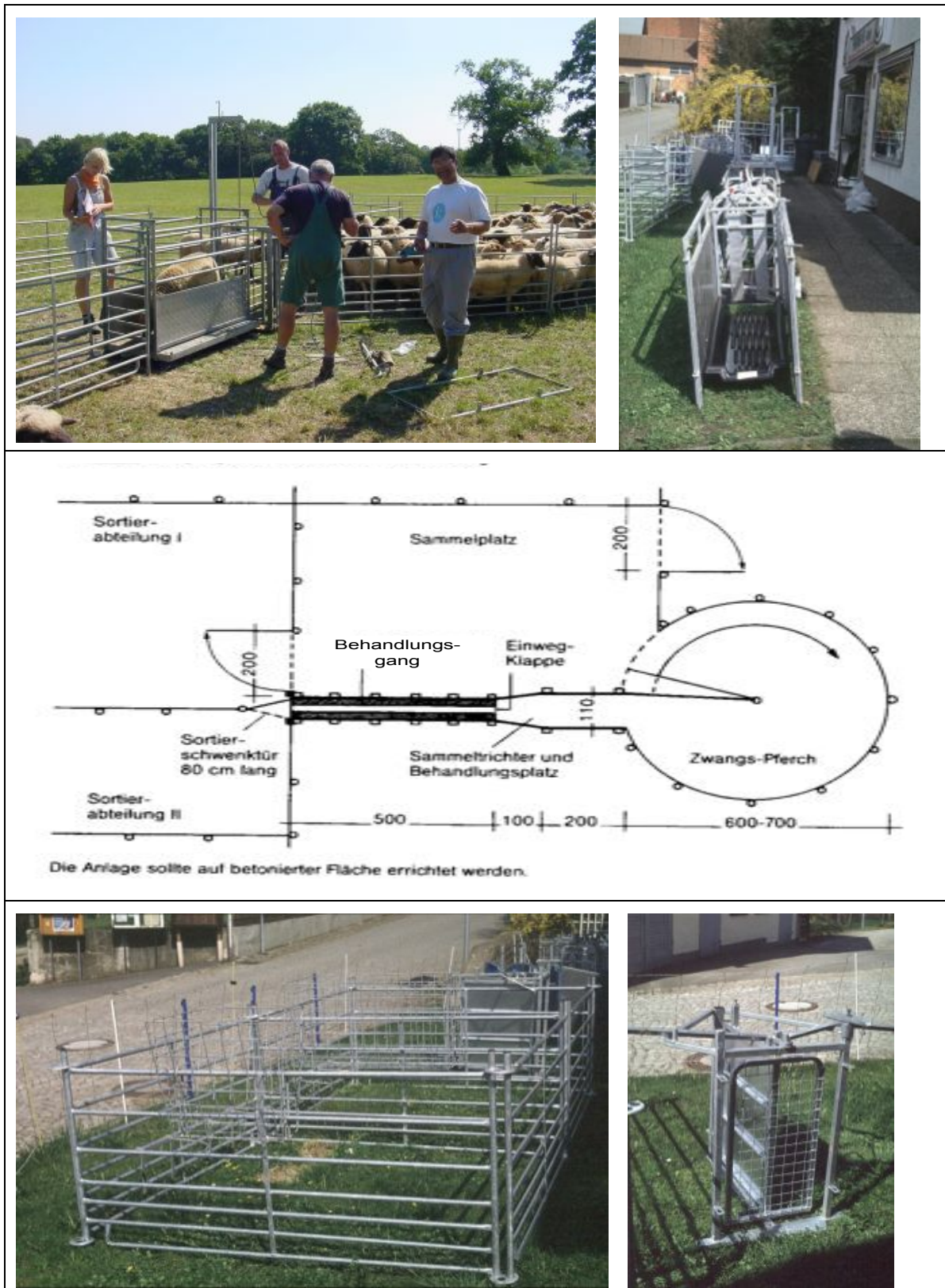
Abb. 45: Behandlungsgang mit Waage (oben, links), Triebgang (oben, rechts), Modell eines Korrels mit Triebgang (Mitte, Korn 2001), Ausstellungsstücke: verzinkte Steckfix-Horden und Selektionstor (unten)
