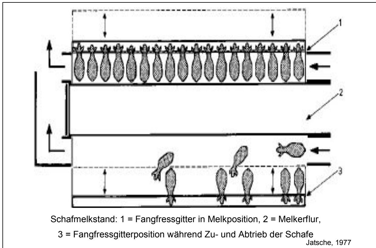
Abb. 99: Schafmelkstand : Ablaufschema des Ein- und Austriebs
