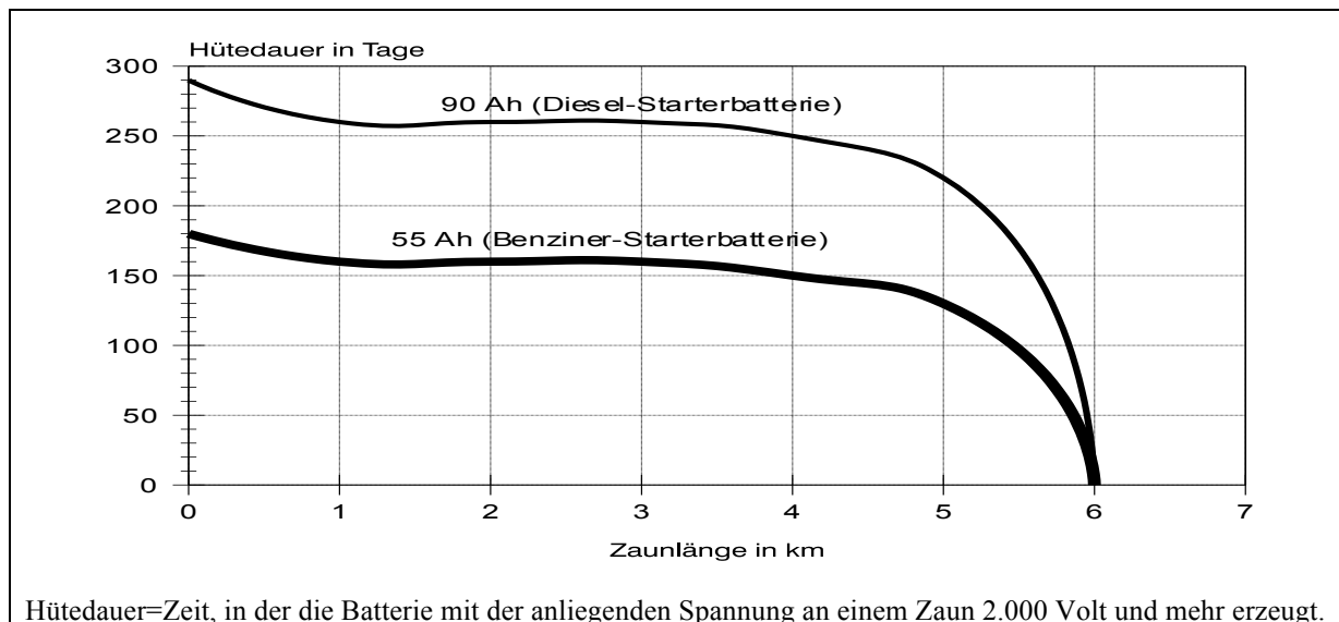
Abb. 35: Die mögliche Hütedauer bei verschiedenen Zaunlängen und Batteriekapazitäten (DLG, in Rahmann, 1998)
