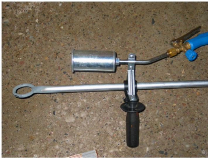
Abbildung 1: Um einen konstanten Abstand zur Oberfläche garantieren zu können wurde eine Halterung mit Fixierung des Brenners entworfen. Die Halterung konnte mit Hilfe eines Schlittens über die Oberflächen bewegt werden.
