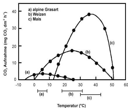
Abbildung 3: Die Temperaturabhängigkeit der Photosyntheseleistung verschiedener Kulturpflanzen
