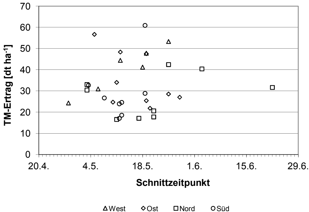
Abbildung 4.2-7: Trockenmasseerträge [dt ha -1 ] des ersten Kleegrasaufwuchses des Jahres 2010 der ökologisch wirtschaftenden Pilotbetriebe in Abhängigkeit vom Schnittzeitpunkt. Differenzierung nach regionaler Zugehörigkeit der Betriebe
