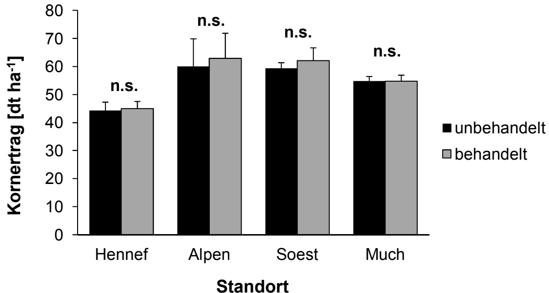
Abbildung 4.3-9: Kornertrag [dt ha -1 ] in Abhängigkeit der Behandlung des Saatgutes mit Pseudomonas chlororaphis . Einfaktorielle Feldversuche der Standorte Hennef, Alpen, Soest und Much. Tukey-Test, \alpha = 0,05
