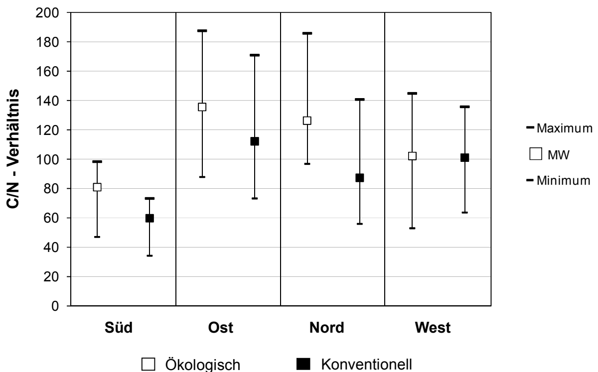
Abbildung 4.3-8: C/N-Verhältnis (dimensionslos) des Stroh im Jahr 2009. Differenzierung nach regionaler Zugehörigkeit und Bewirtschaftungsweise der Betriebe. Dargestellt sind das jeweilige Minimum, Maximum und arithmetische Mittel.
